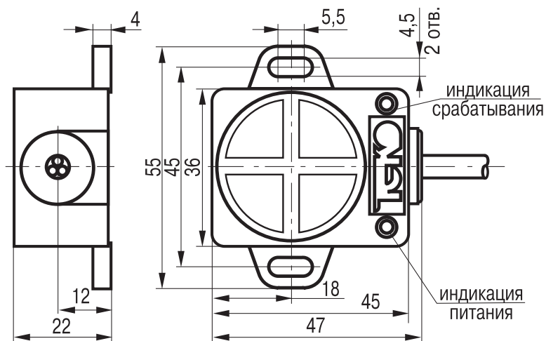
Габаритный чертеж
